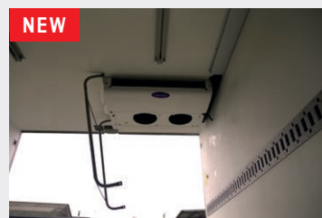
Protezione dell'evaporatore apribile
