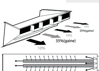
Convogliatore AirEfficient-C Evo Altezza - 70mm per passaggio pallet alti
